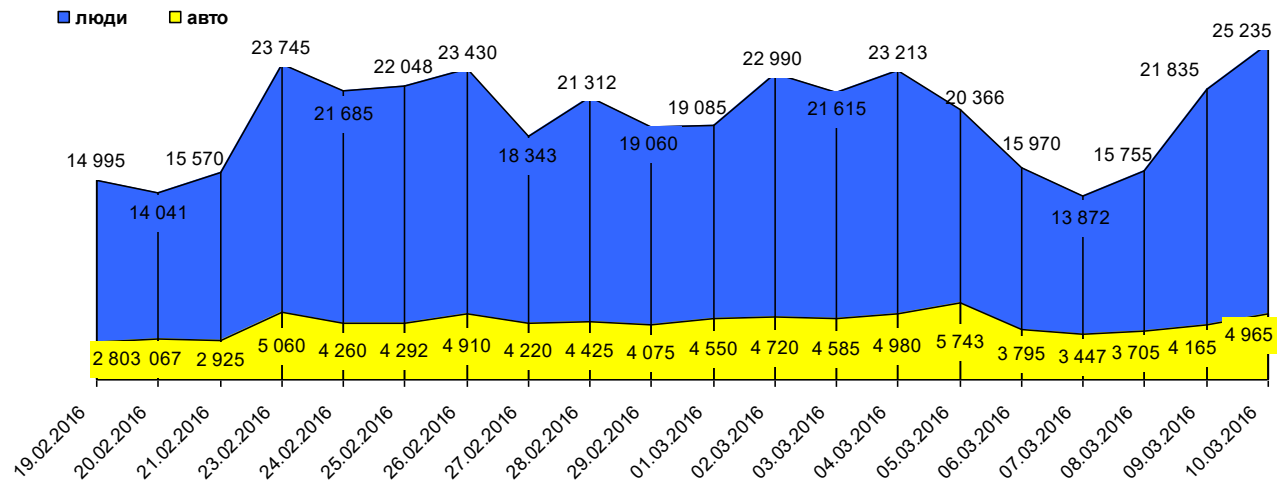
Мал. 5 – Пасажиро-транспортний потік в контрольних пунктах в'їзду-виїзду на лінії розмежування в зоні проведення АТО.
